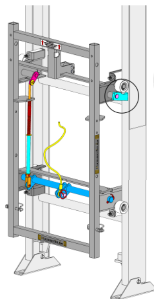
Patin parachute FERME Chariot bloqué
