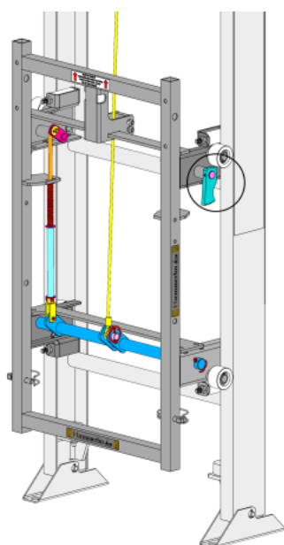
Patin parachute OUVERT Chariot libéré
