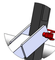
Détail du verrouillage
