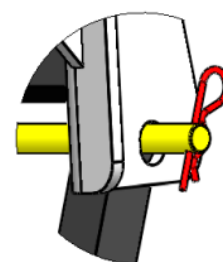
Détail du verrouillage
