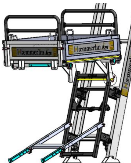
Détail du verrouillage
