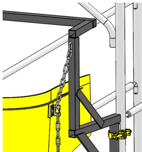
Détail de l'accrochage des chaînes
