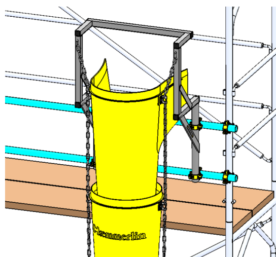
Installation en façade d'échafaudage
