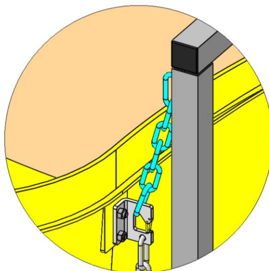
Détail de l'accrochage des chaînes
