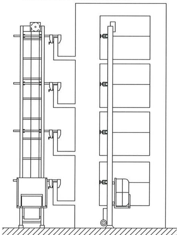
ECHELLE PERPENDICULAIRE AU BATIMENT Ancrage sur le mur ou la balustrade de balcon au moyen du serre-joint d'embrasure
