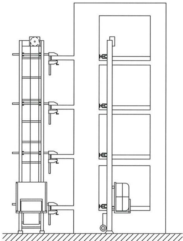
ECHELLE PARALLELE AU BATIMENT Echelle directement en appui contre la rampe du balcon et ancrée au moyen de crampons
