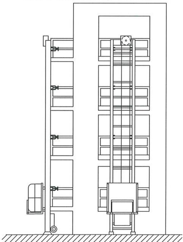
ECHELLE PARALLELE AU BATIMENT Echelle directement en appui contre la rampe du balcon et ancrée au moyen de crampons
